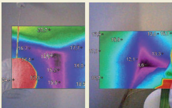
Zřetelně viditelné studené kouty místnosti v pohledu termokamery, ideální místo pro plošnou aplikaci ETERNAL In Thermo .
