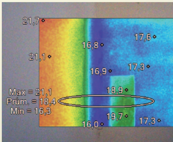
Termofotografie ukazuje změnu povrchové teploty stěny (zelený obdélník) v místě aplikovaného vzorku barvy ETERNAL IN Thermo .
